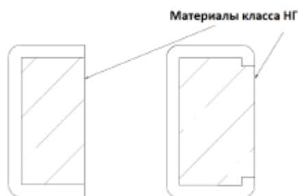
Рисунок Г.5 – Пример заполнения пространства в сечении конструкции
