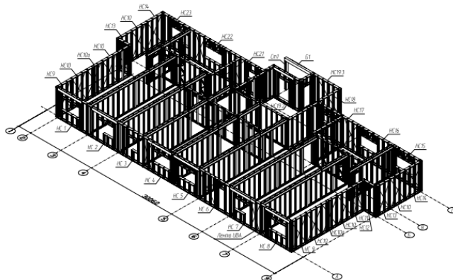
Рисунок 7.7 – Каркасное здание из ЛСТК
