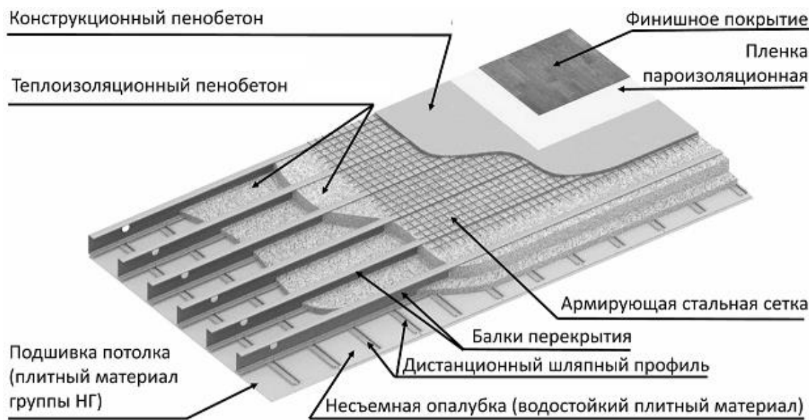
Рисунок 11.6 – Балочное перекрытие с жестким диском из армированного конструкционного пенобетона
