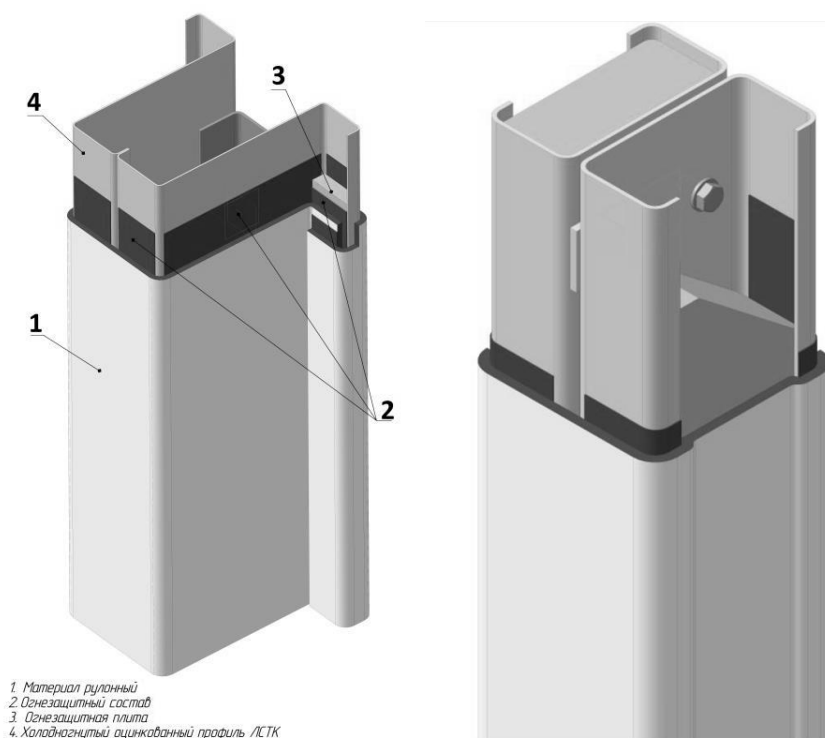
Рисунок Г.6 – Пример технического решения с заполнением
