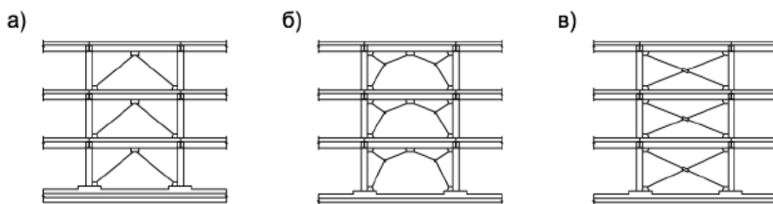
а) – треугольные; б) – порталные; в) – крестовые Рисунок 7.2 – Схемы сквозных вертикальных связей
