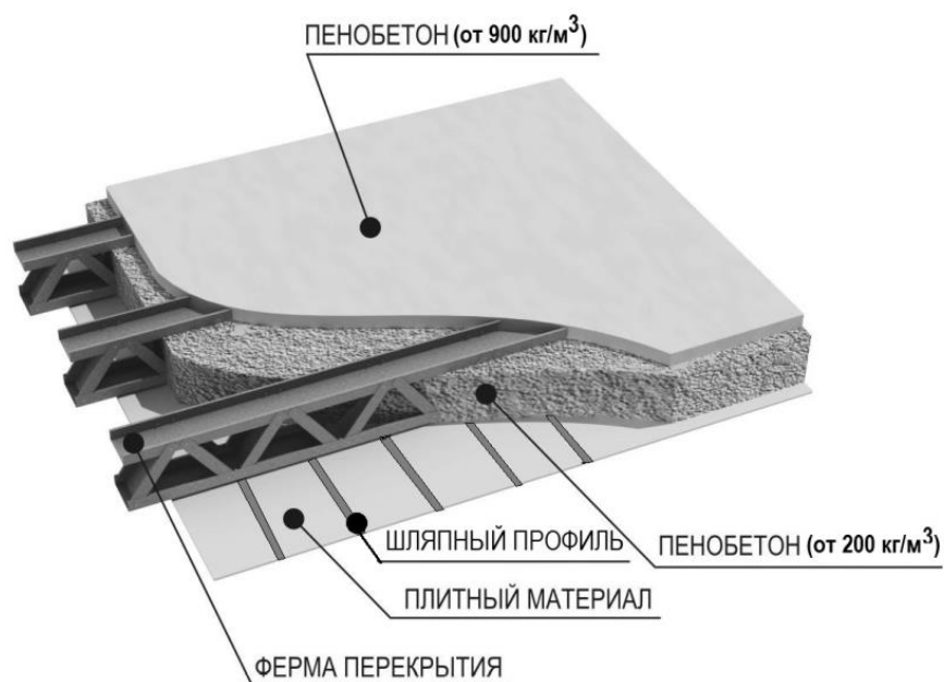
Рисунок Г.7 – Пример огнезащиты конструкций жилых домов из ЛСТК: а – внутренняя стена; б – перекрытие
