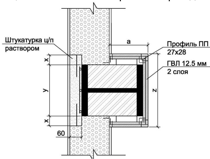
Рисунок Г.1 – Примерная схема облицовки стальной колонны, находящейся в составе ограждающей конструкции, листовыми материалами типа ГКЛ, ГВЛ в один слой (ограждающая стеновая конструкция показана условно)
